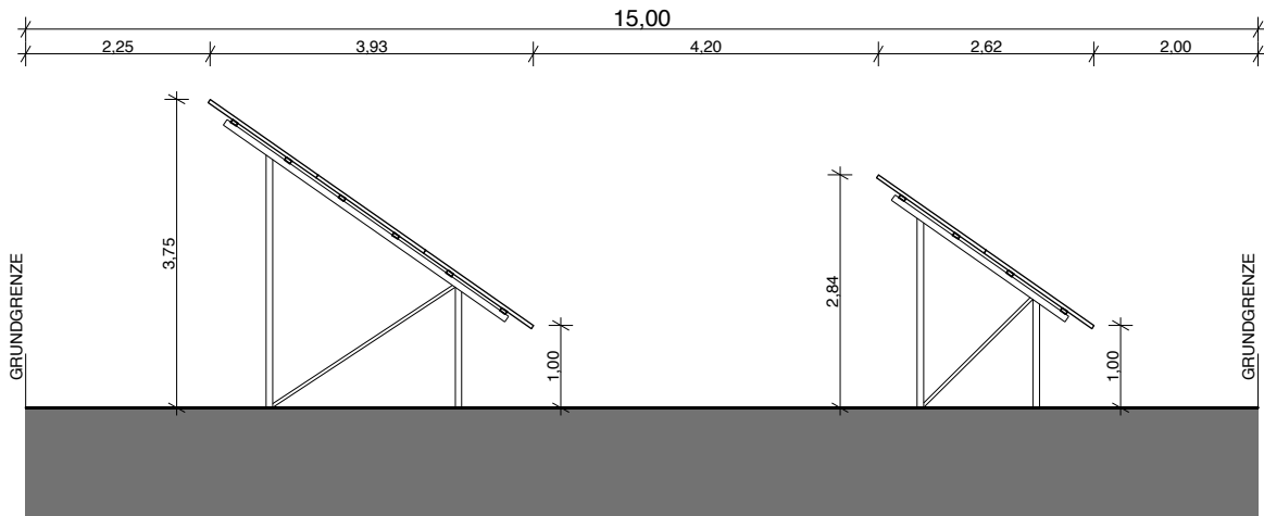
Schnitt M 1:100
