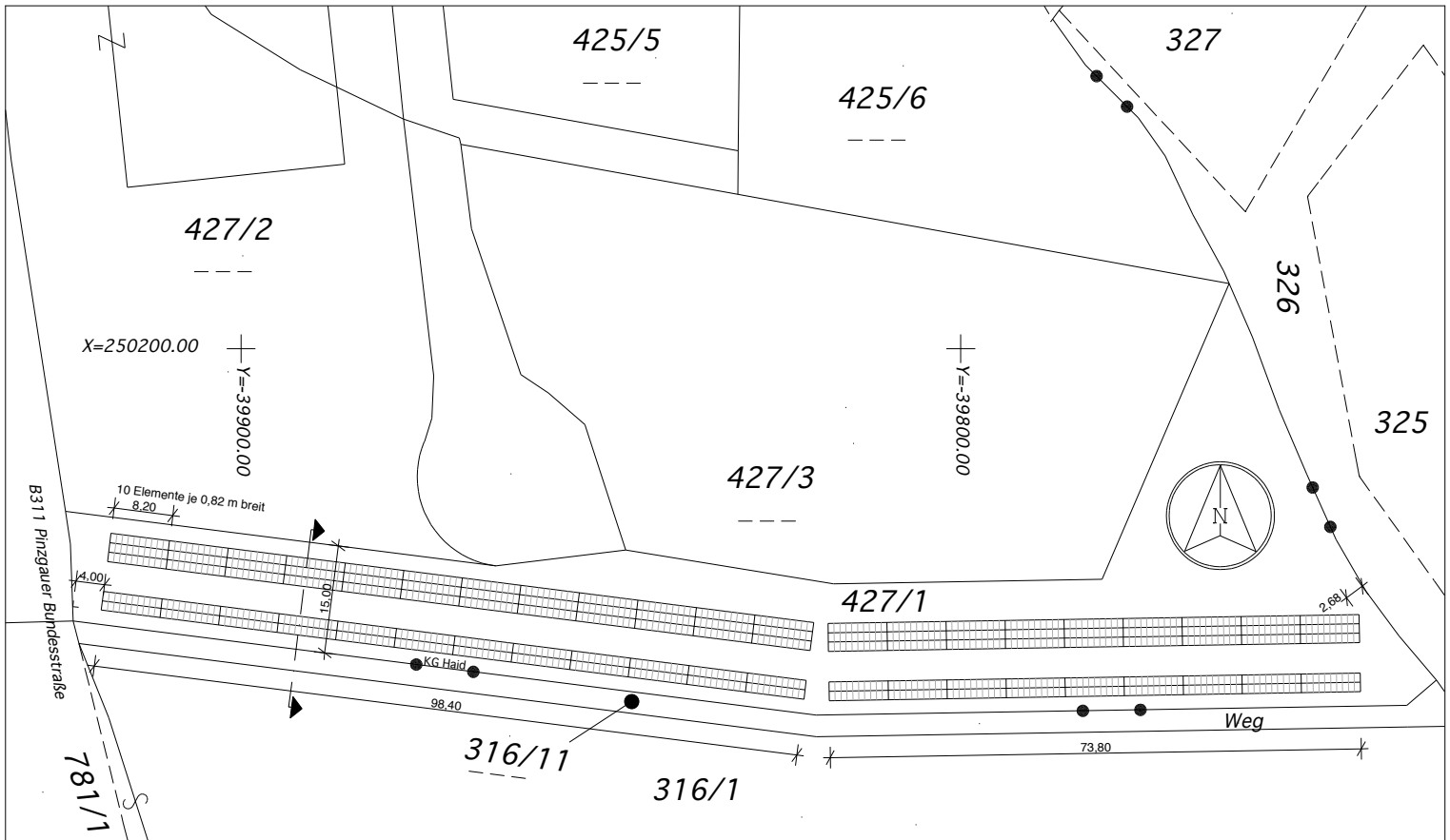
Lageplan M 1:1000
